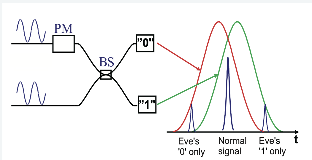
FIGURE 4 – Probabilité de détection d'un photon en fonction du temps pour les deux récepteurs
