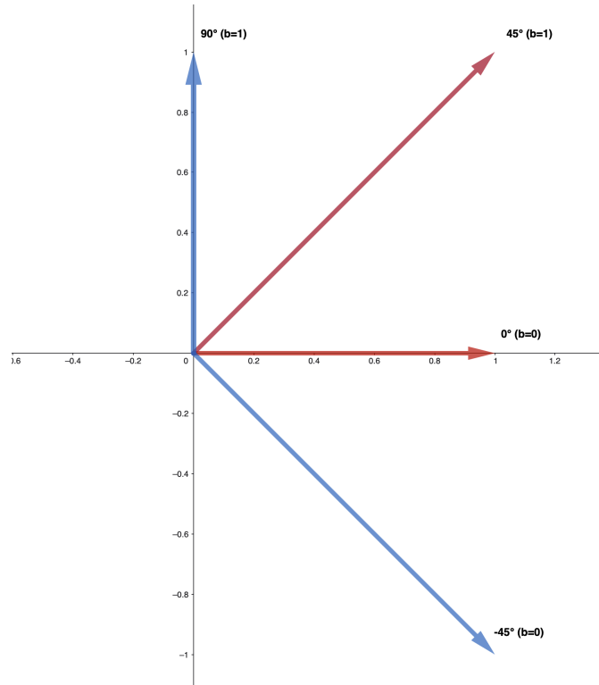
FIGURE 3 – Représentation des ensembles de vecteurs.
