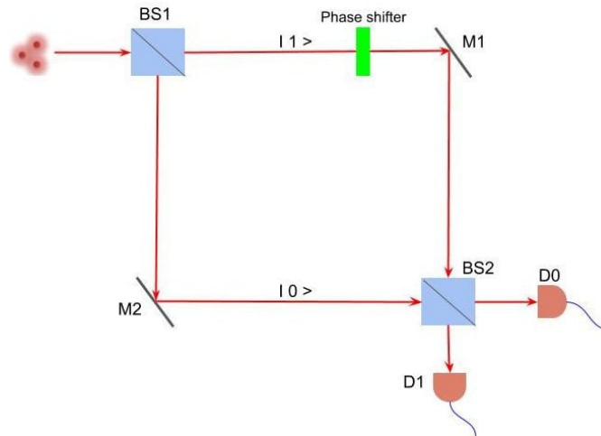
FIGURE 2 – Interféromètre de Mach-Zehnder.
